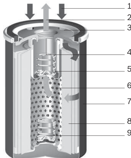
Sección de filtro
