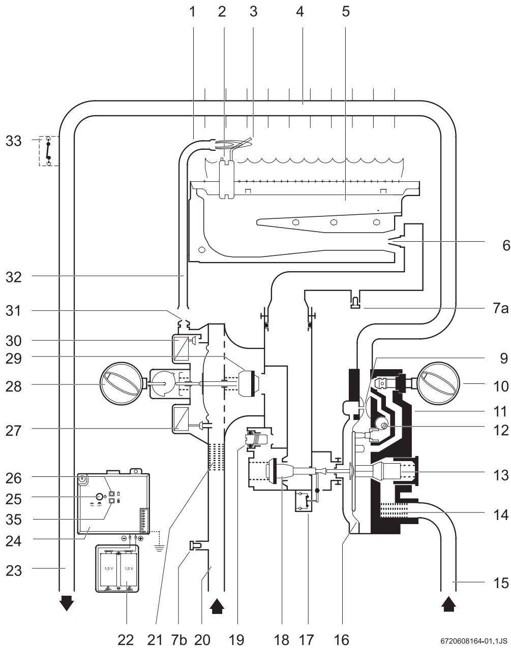
Fig. 2 Esquema técnico
