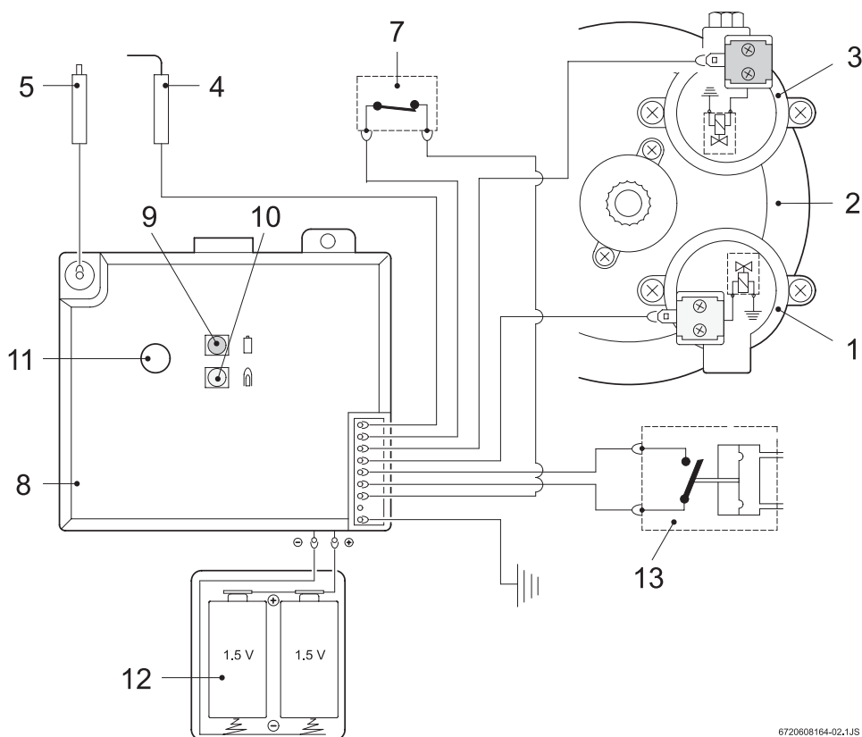
Fig. 3 Esquema eléctrico
