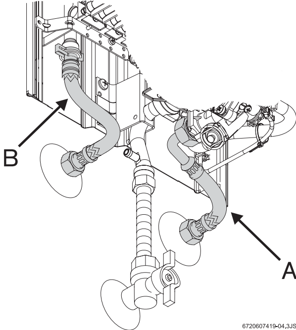
Fig. 7 Conexión del agua
